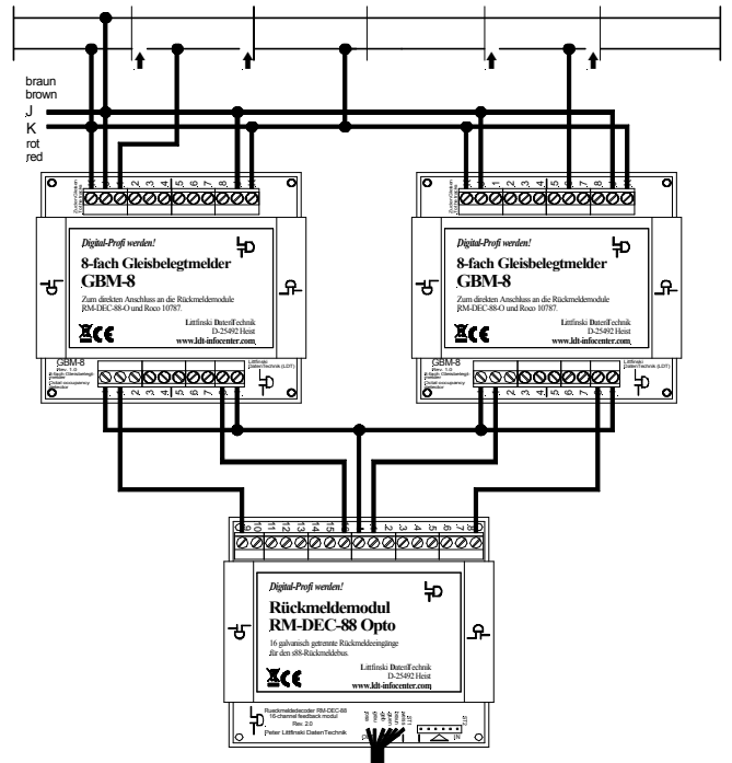
Abbildung 4: Auch das 16-fach Rückmeldemodul RM-DEC-88-O für den s88-Rückmeldebus, kann durch zwei GBM-8 um die Funktion „Gleisbelegtmeldung“ erweitert werden.
